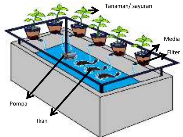
Gambar 2. Desain instalasi akuaponik dan lanscape lahan budidaya yang diterapkan.
